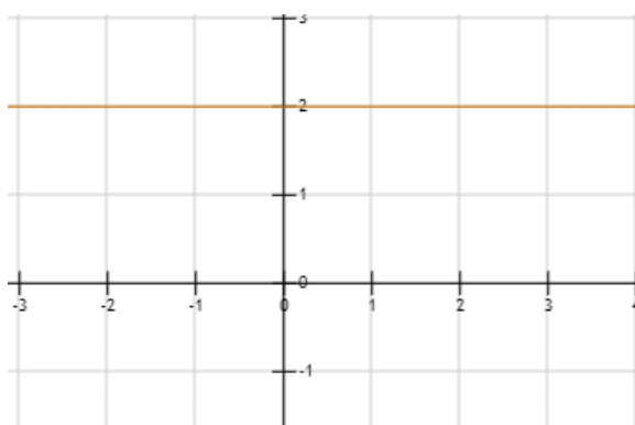
Imagen 38: Gráfica función constante.
