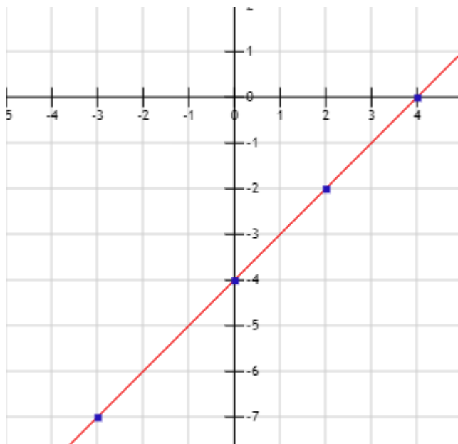
b) GRÁFICA 2
