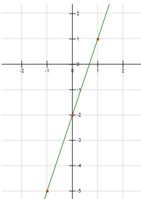
Imagen Nº 10. Gráfica. Fuente: Imagen de Elaboración Propia
