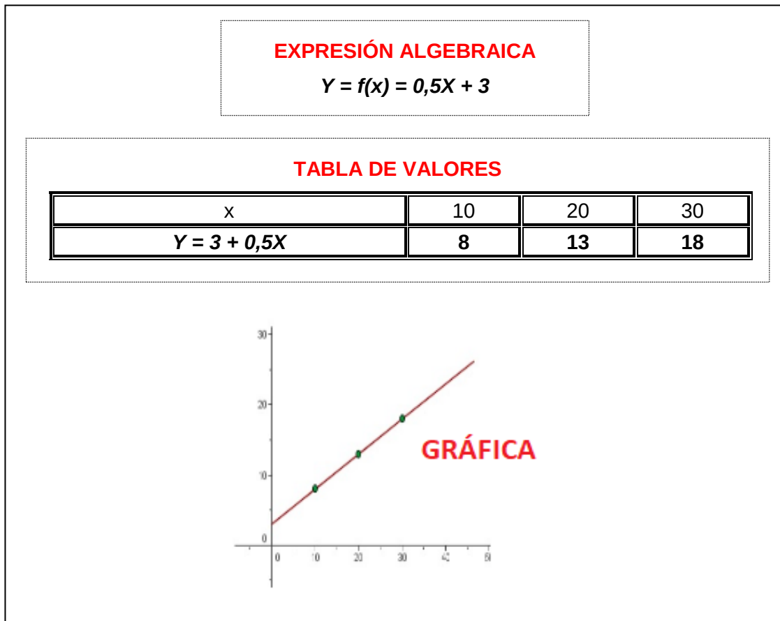
Imagen Nº 1. Representación de Funciones. Fuente: Imagen de Elaboración Propia
