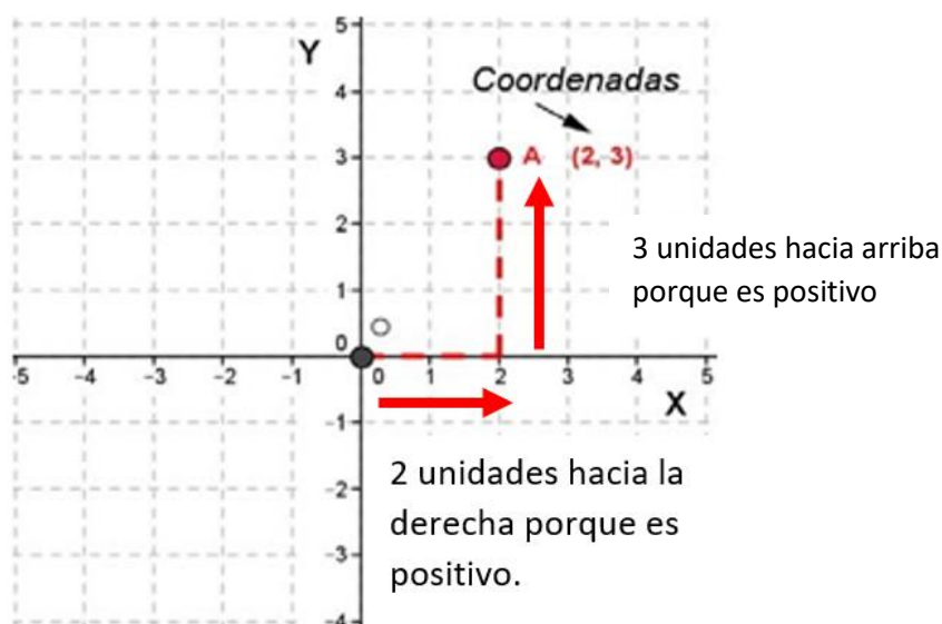
Imagen N° 5. Coordenadas. Fuente: Imagen de Elaboración Propia
