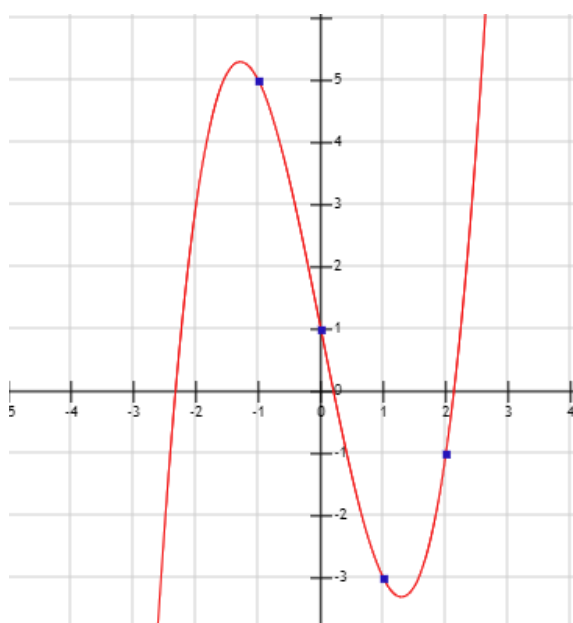
a) GRÁFICA 1
