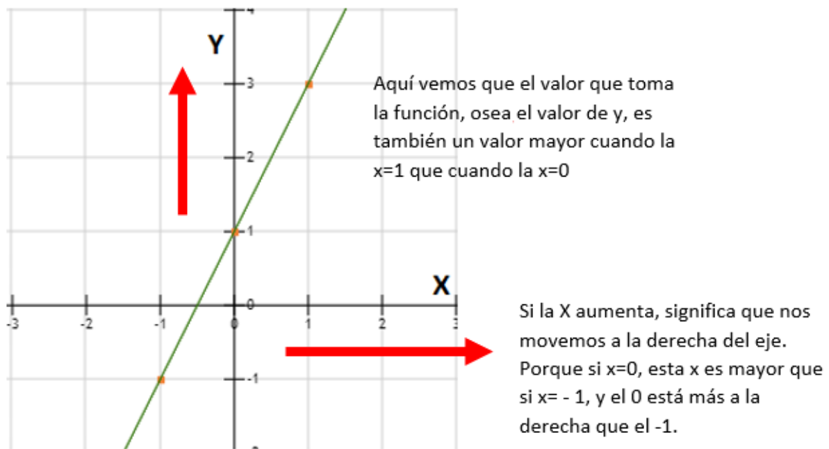
Imagen N° 15. Gráfica Creciente. Fuente: Imagen de Elaboración Propia
