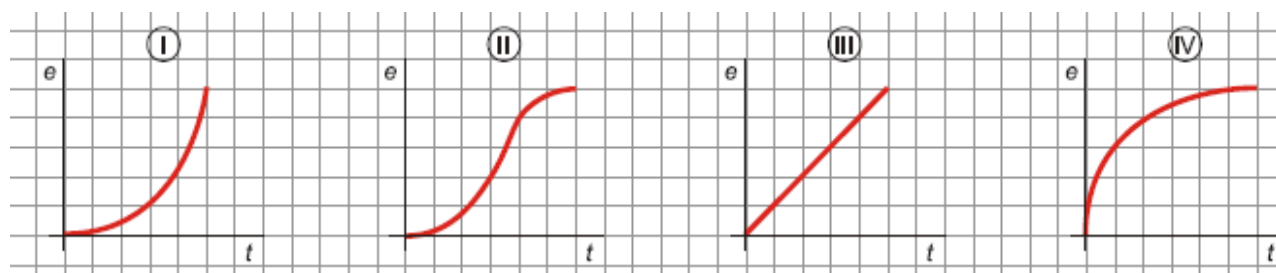
Imagen 23: Gráficas.
