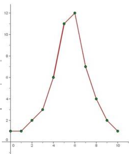
Imagen Nº 13. Gráfica y Tabla de Datos. Fuente: Imagen de Elaboración Propia
