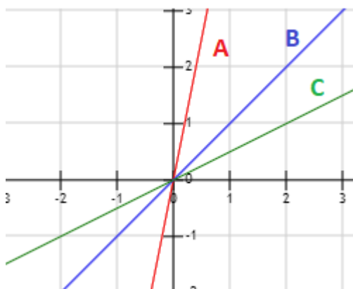
Imagen 33: Funciones lineales.
