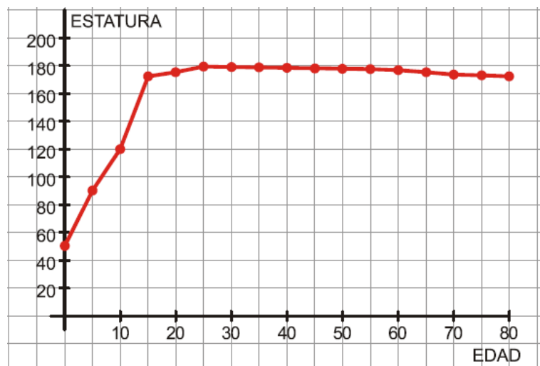
Imagen 27: Gráfica.
