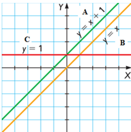
Imagen 39: Gráficas de funciones
