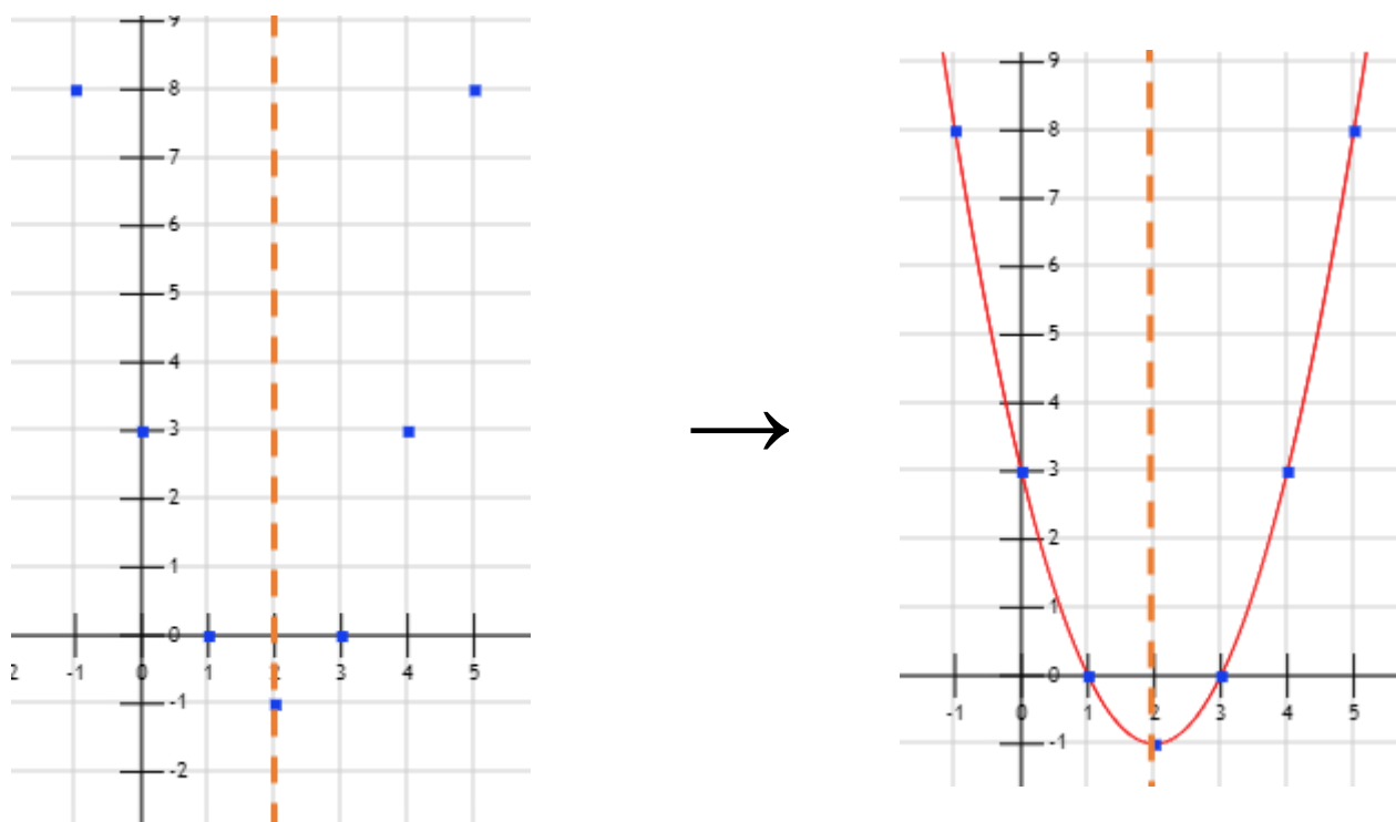
Imagen 45: Representación de una función cuadrática.
