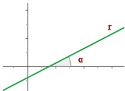
Función CRECIENTE m > 0
