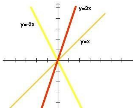
Imagen 28: Gráfica funciones lineales
