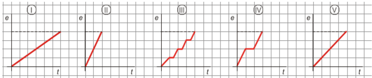
Imagen 26: Gráficas.
