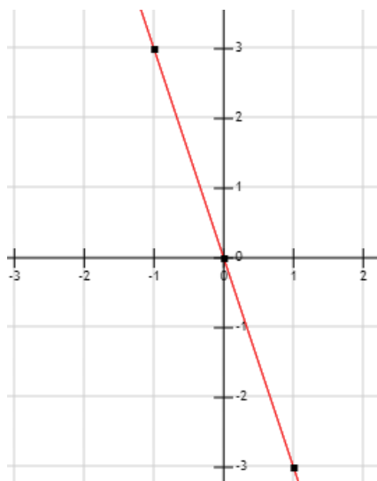
Imagen 34: Función lineal.
