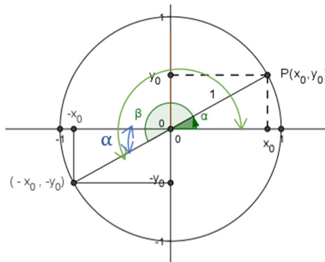
Imagen 12: Relación entre ángulos del primer y tercer cuadrante. Fuente: Propia.
