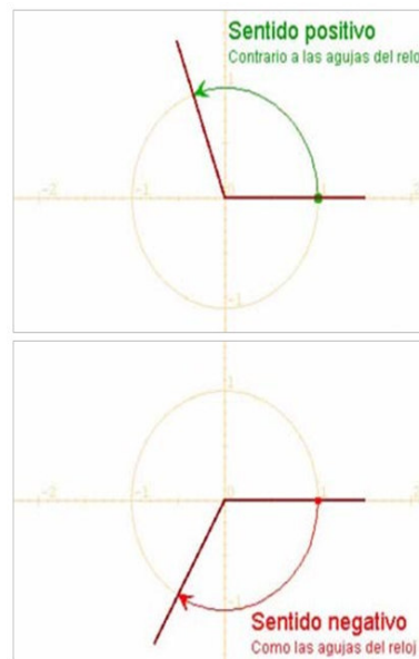
Imagen 4: Sentidos de los ángulos.
